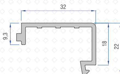
Louvre Clip 41101 - 18000
