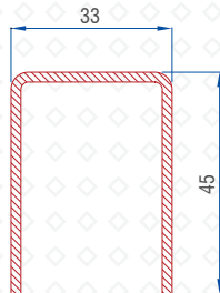
Mega Sash Reinforcement 2.0mm : 56016 - 20047
