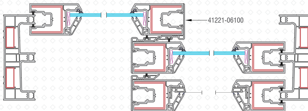
SEC A-A
