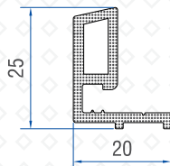
Mesh Adaptor (Alm) 50502 - 11041
