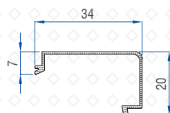
I-39 Louvre Clip(Alm) 50502-11056
