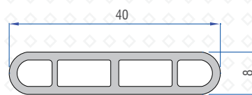
Louvre Blade 41101 - 18100
