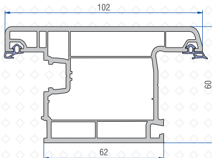
Door Sash Profile 41101 - 14000
