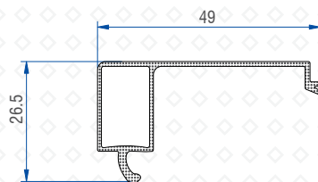
Fixed Louver Clip (Alm) 50502 - 11038
