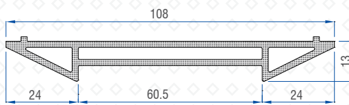
New 3 -Track Coupler(Alm) 50502-11057
