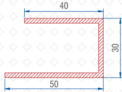
Door Sash Reinforcement 1.5mm : 56016 - 15012
