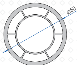
Pipe Profile 40104 - 03000
