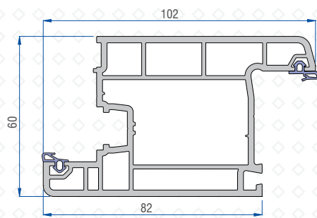
Inward Opening Door Sash Profile 41101-14100
