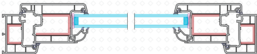
SEC A-A
